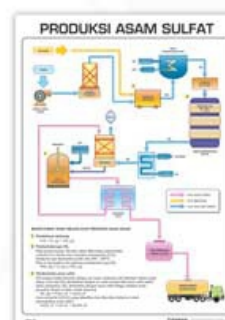
Carta Produksi Asam Sulfat | VCK 25
