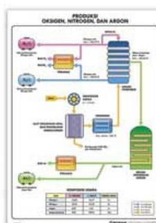
Carta Produksi Oksigen, Nitrogen, dan Argon | VCK 24
