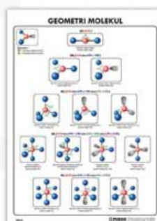
Carta Geometri Molekul | VCK 13
