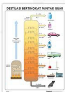
Carta Destilasi Bertingkat Minyak Bumi | VCK 12
